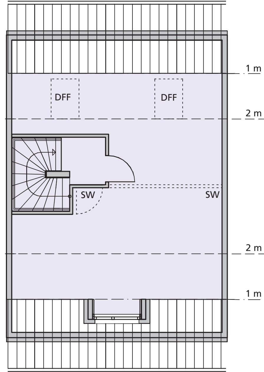
Dachgeschoss
