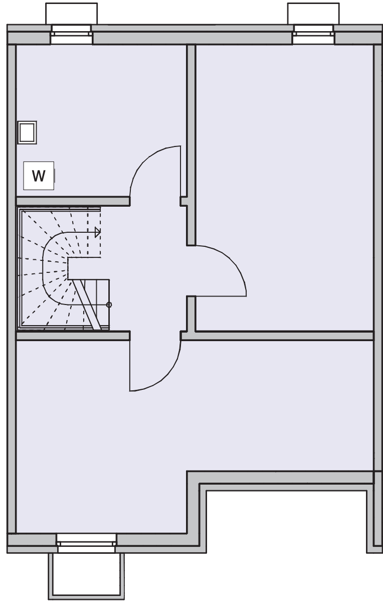
Untergeschoss
